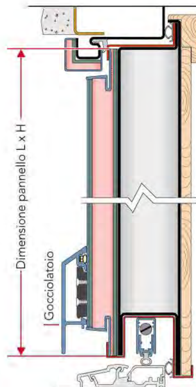
Particolare aletta cingivetro su pannelli a vetri delle collezioni A Filo e Emotion .
