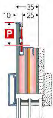
Tipo EM 35 Up 0.86 W/m²k Rw 33 dB Kg 18,0 m²
