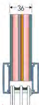
Tipo TP 36 Up 0.86 W/m²k Rw 33 dB Kg 20,0 m²
