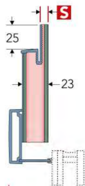
Tipo KE 23 Up 1.2 W/m 2 k Kg 10,5 m 2
