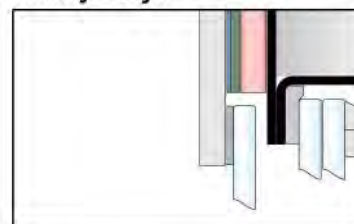
Particolare vetro satinato temprato sp. 4 mm, inserito su pannelli a vetri delle collezioni Infinity e Style .
