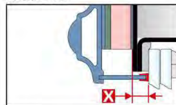
Particolare vetro satinato temprato sp. 4 mm, inserito su pannelli a vetri delle collezioni Infinity e Style .
