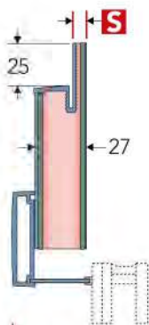
Tipo KE 27 Up 0.98 W/m 2 k Kg 11,0 m 2
