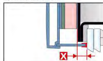
Particolare aletta cingivetro su pannelli a vetri della collezione Novecento .
