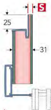
Tipo KE 31 Up 0.81 W/m 2 k Kg 11,5 m 2
