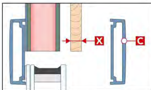
Cornice lato interno per pannelli Plus-Mix. Su richiesta.
